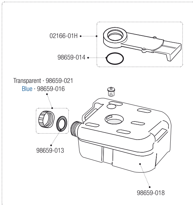
Bi-Pot 1520
